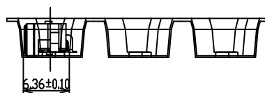
SECATION A-A
