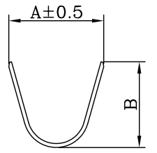
SEC A-A'
