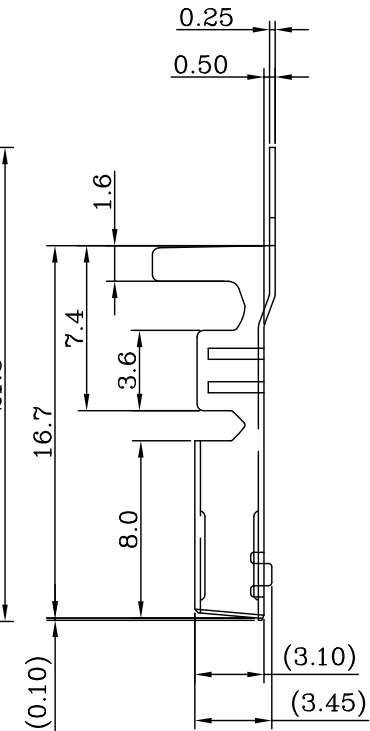
SEC A-A'
