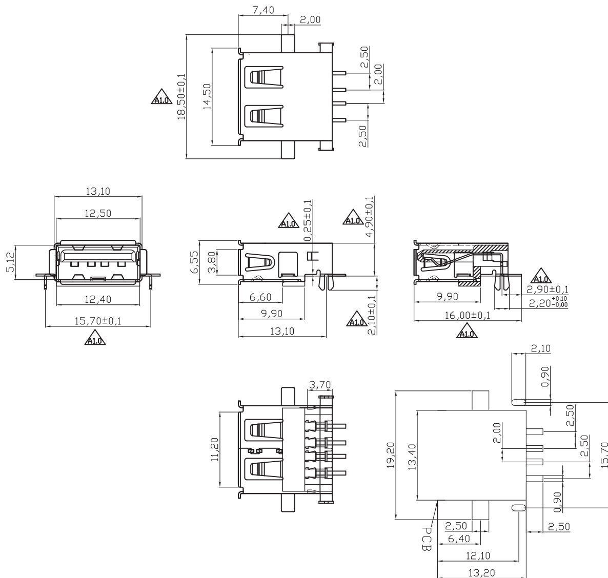
P.C.B. LAYOUT
