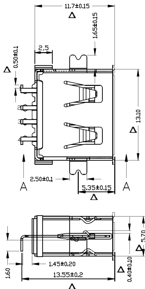
SECTION A-A
