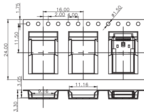
① 產品入載帶示意圖
