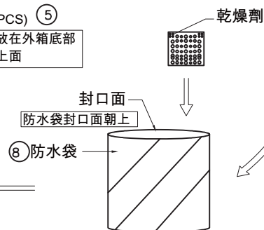
④ 7盤產品入防水袋示意圖
