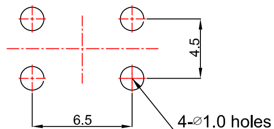
P.C.B LAND PATTERN
