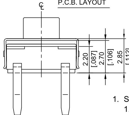
(SCALE 8:1) P.C.B. LAYOUT
