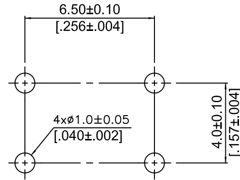
(SCALE 8:1) P.C.B. LAYOUT
