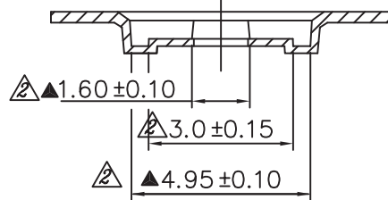
A-A Section
