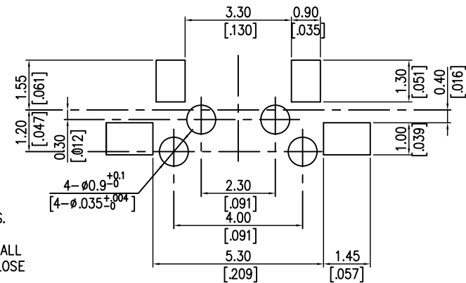
P.C.B. LAYOUT
