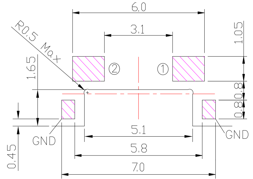
P.C.B LAYOUT
