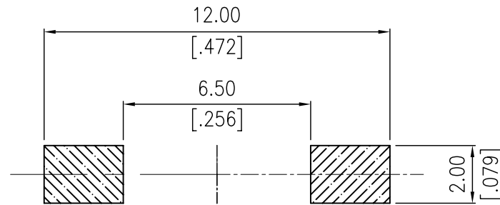
P.C.B. LAYOUT
