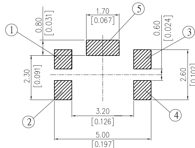
P.C.B. LAYOUT
