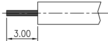
CABLE STRIPPING DIM.
