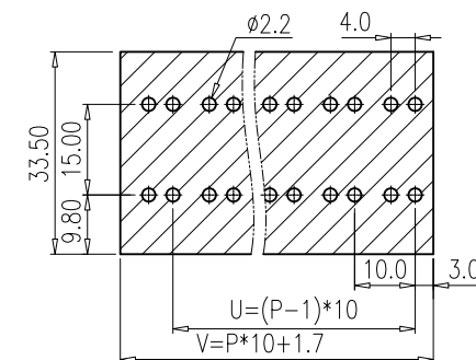
PCB LAYOUT(S=1:1)
