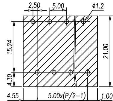
P.C.B. LAYOUT(REF)
