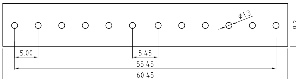
P.C.B. LAYOUT
