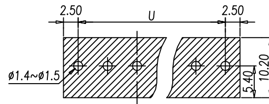
P.C.B. LAYOUT(REF)
