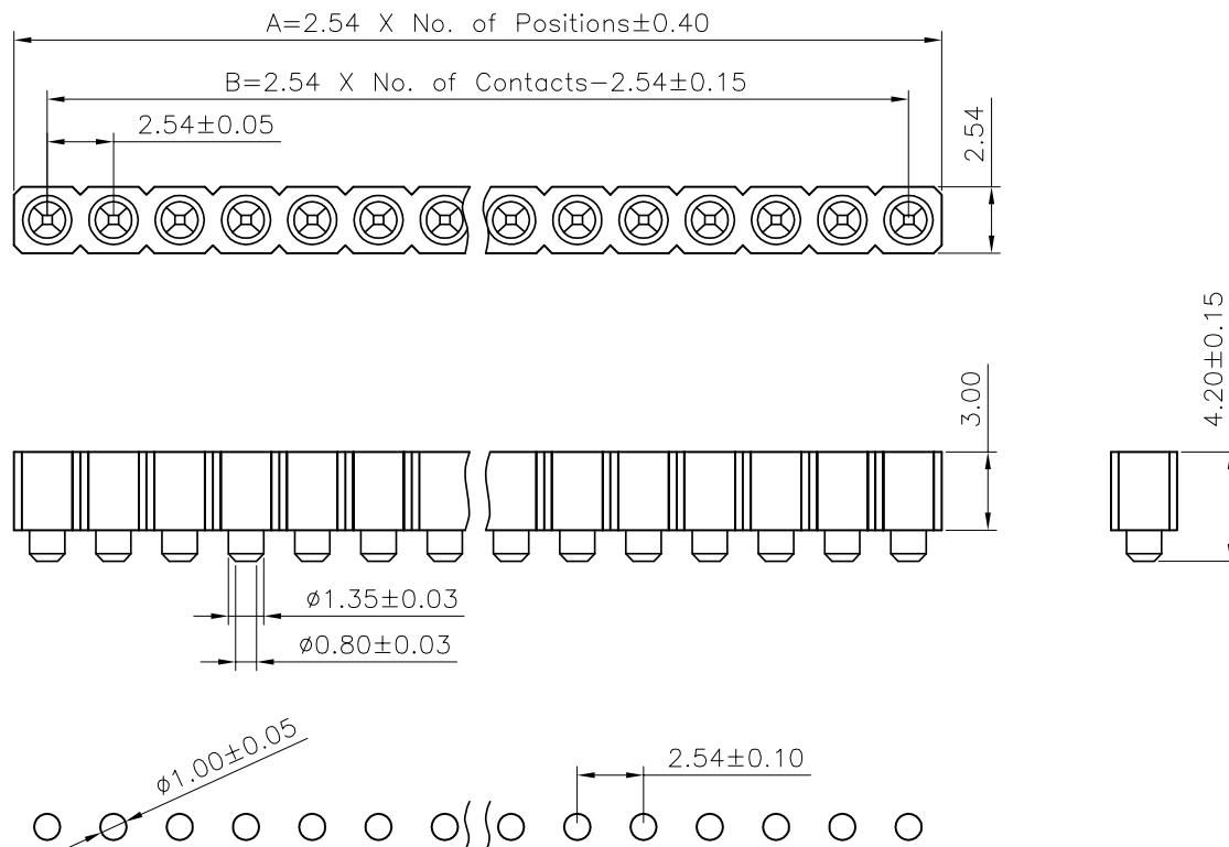
P.C.B LAYOUT
