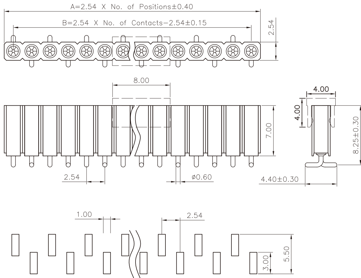
P.C.B LAYOUT
