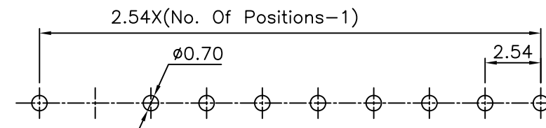
P.C.B Layout
