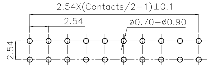
P.C.B LAYOUT
