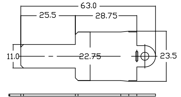
SONY 接觸片(鍍) 材質/MATERIAL: 鋼/Steel 電鍍/PLATING: 鍍/Nickel
