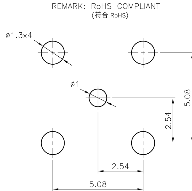
P.C.B. LAYOUT (印刷电路板配置)
