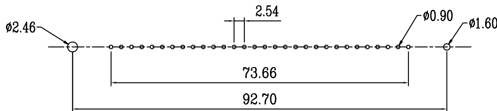
P.C.B. layout
