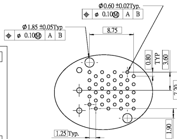
細部放大圖 D 比例 3 : 1
