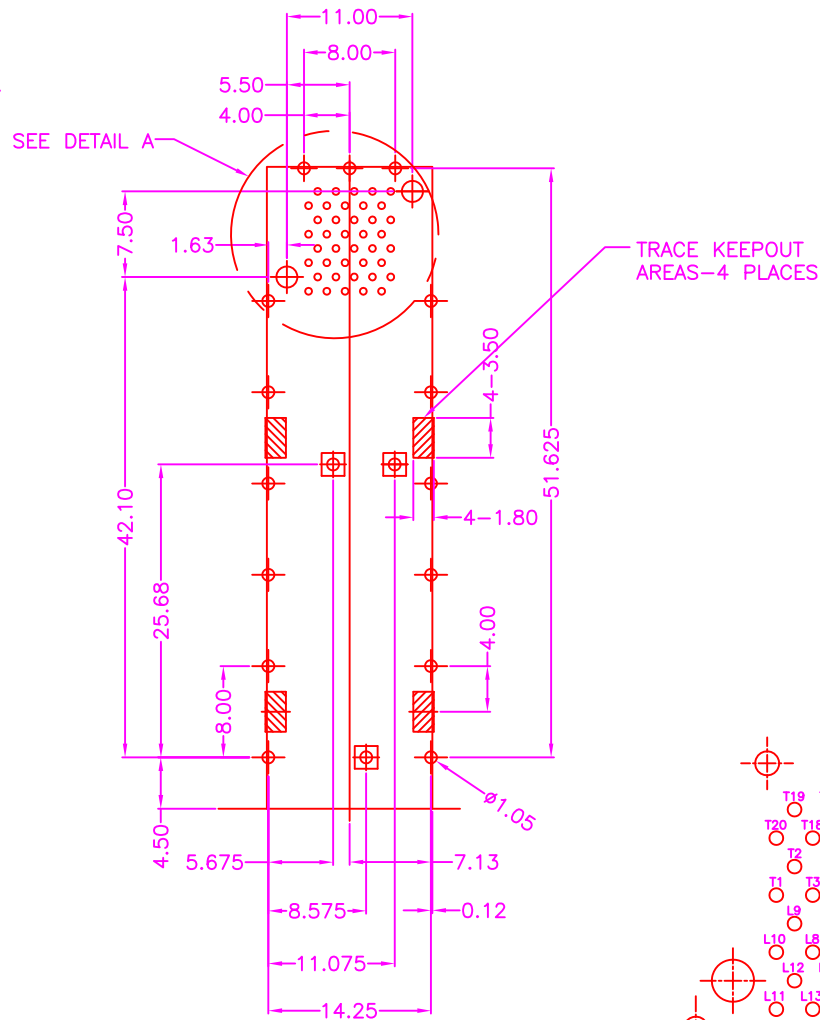
P.C.B LAYOUT TOP VIEW \pm 0.05
