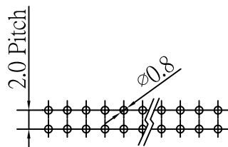
P.C.Board Layout
