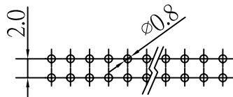
P.C.Board Layout
