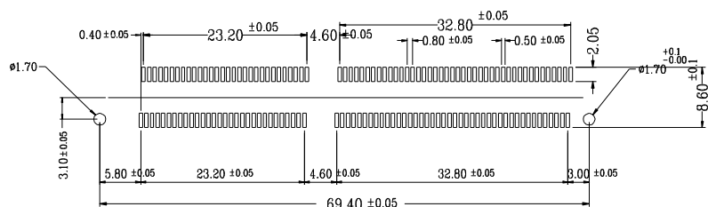
P.C.B. Layout
