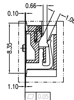
DETAIL:A SCALE:2:1
