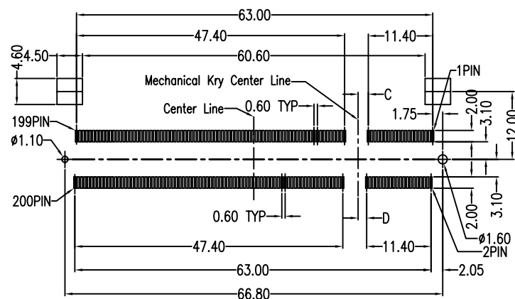
P.C.B LAYOUT
