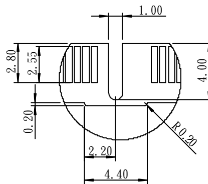
B (4 : 1)
