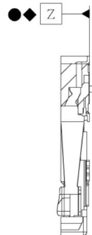
A-A (2 : 1)
