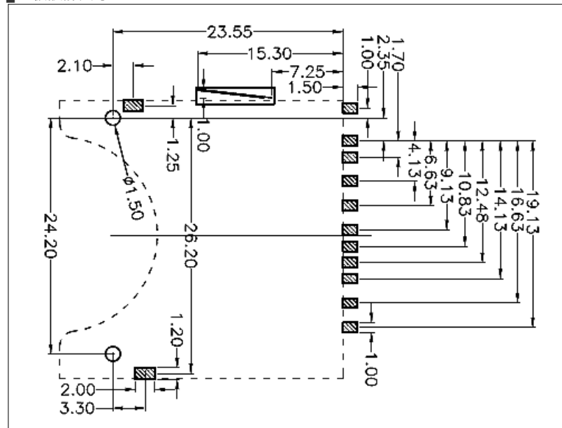
基板設計尺寸
