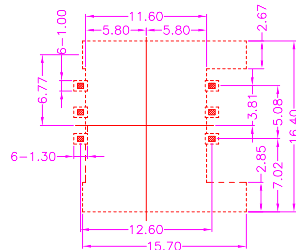
P.C.B LAYOUT TOP VIEW \pm 0.05
