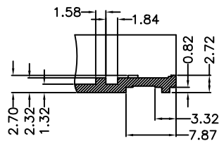
SECTION A-A (scale: 2:1)
