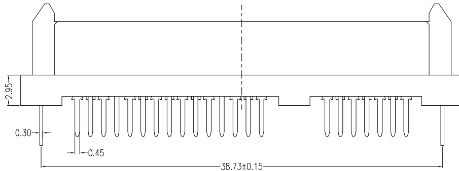
SECT A-A
