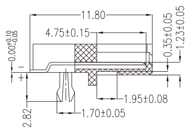
SECT A-A
