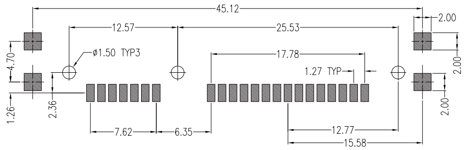
P.C.B Layout
