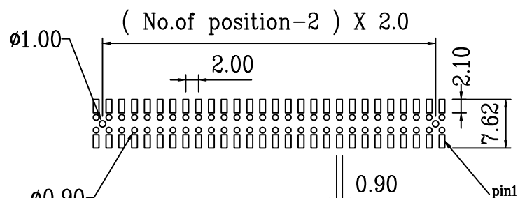
P.C.B.layout
