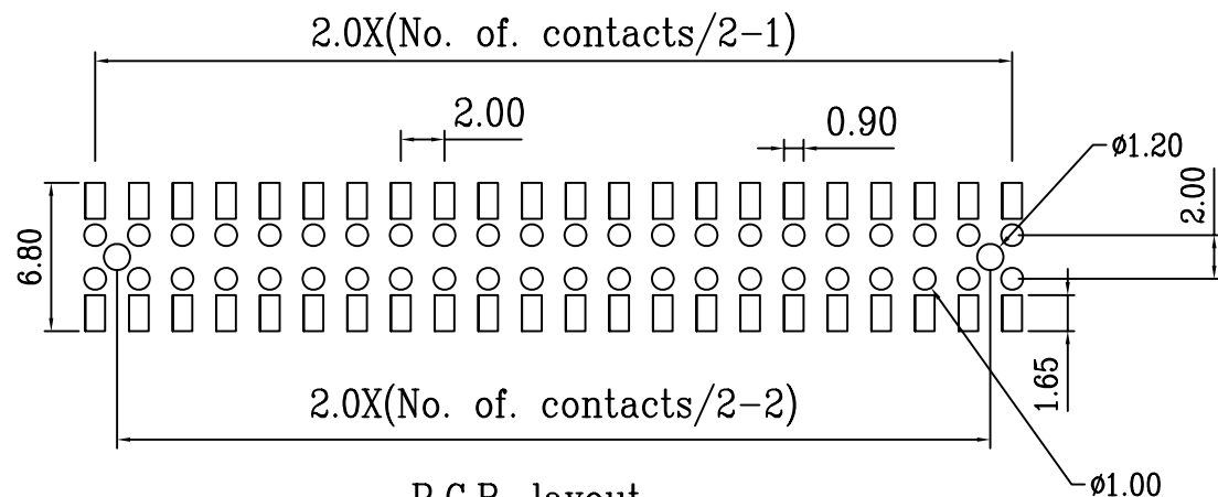
P.C.B. layout
