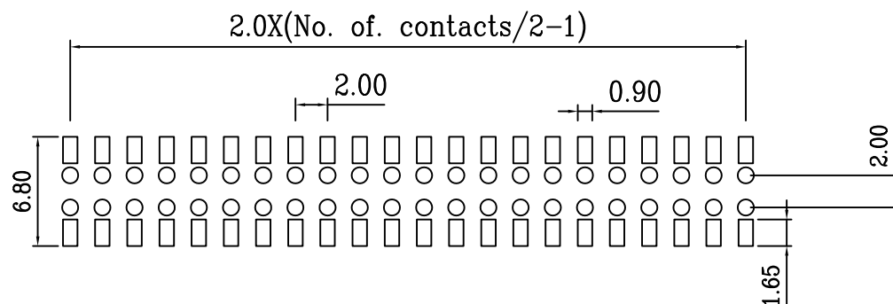
P.C.B. layout
