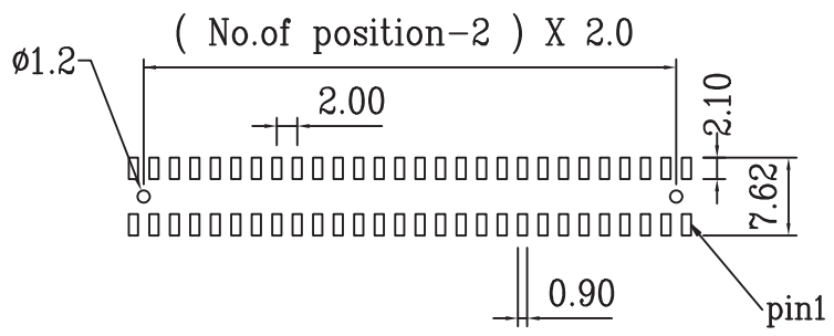
P.C.B.layout
