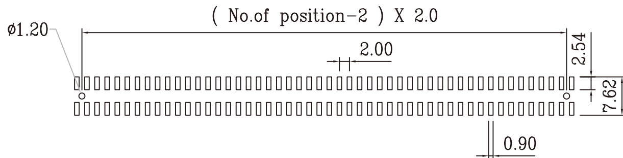
P.C.B.layout
