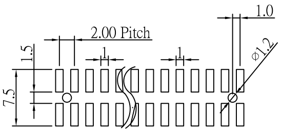
P.C.Board Layout
