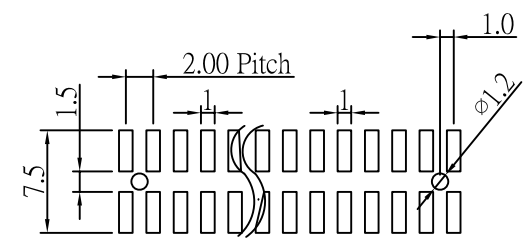
P.C.Board Layout
