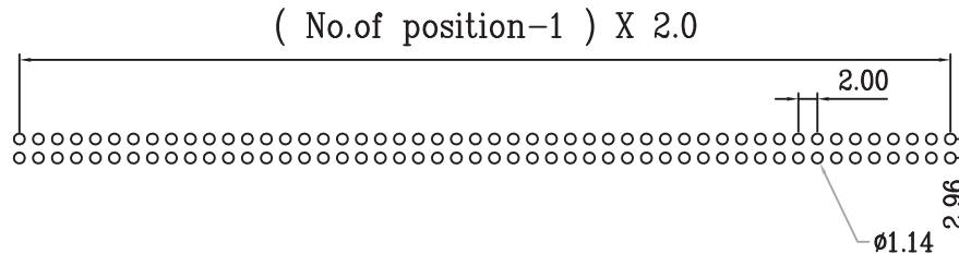
P.C.B.layout
