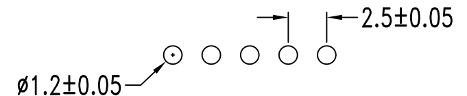
P.C.B. Hole Dimensions
