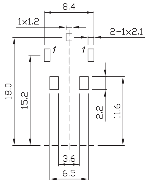
P.C.B LAYOUT(±0.1) (BOTTOM VIEW)
