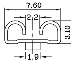
SEC. A-A
