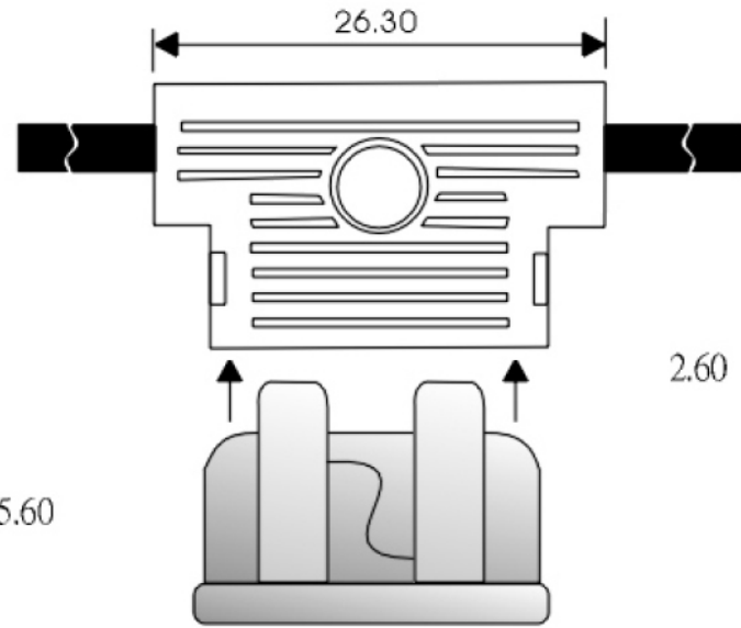
(保險絲) Fuse
